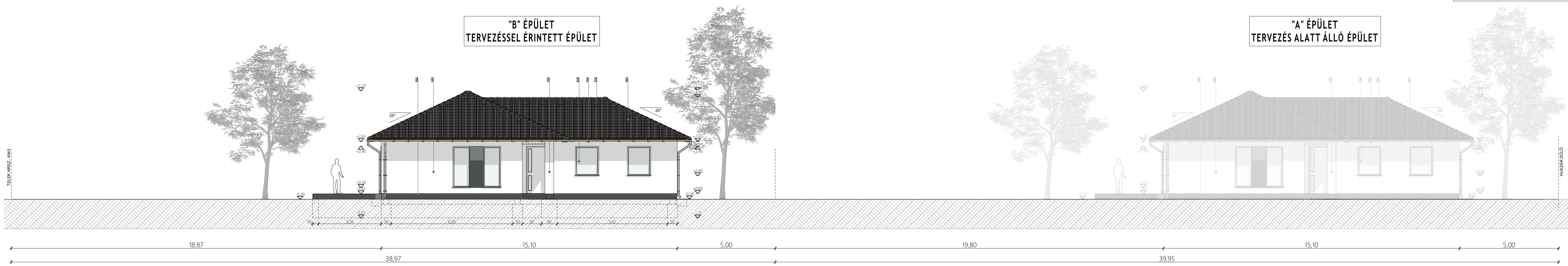
DÉLI HOMLOKZAT(M=1:100)
